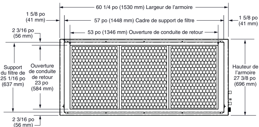
Figure 5. Dimensions physiques B6TM pour les installations horizontales
