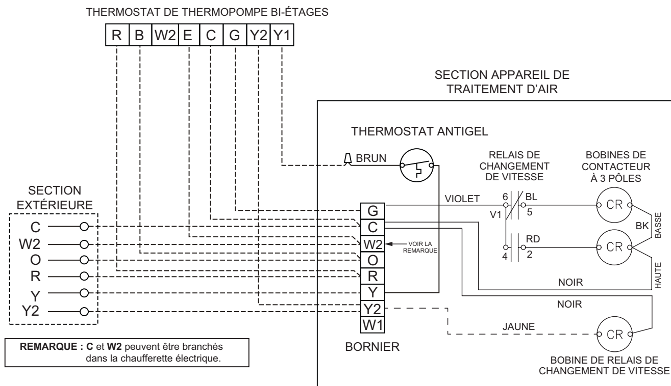
BRANCHEMENTS TYPQUES DU THERMOSTAT DE LA THERMOPOMPE
