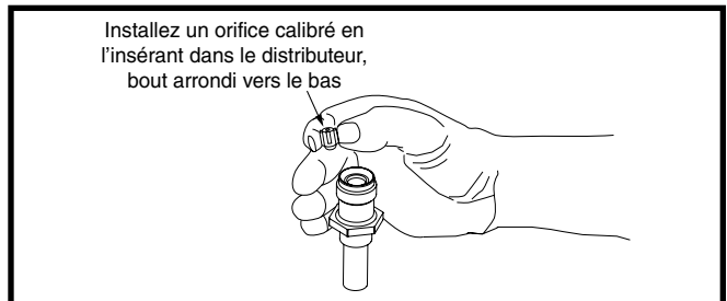
Figure 4. Insertion de l'orifice d'étranglement dans le corps du distributeur
