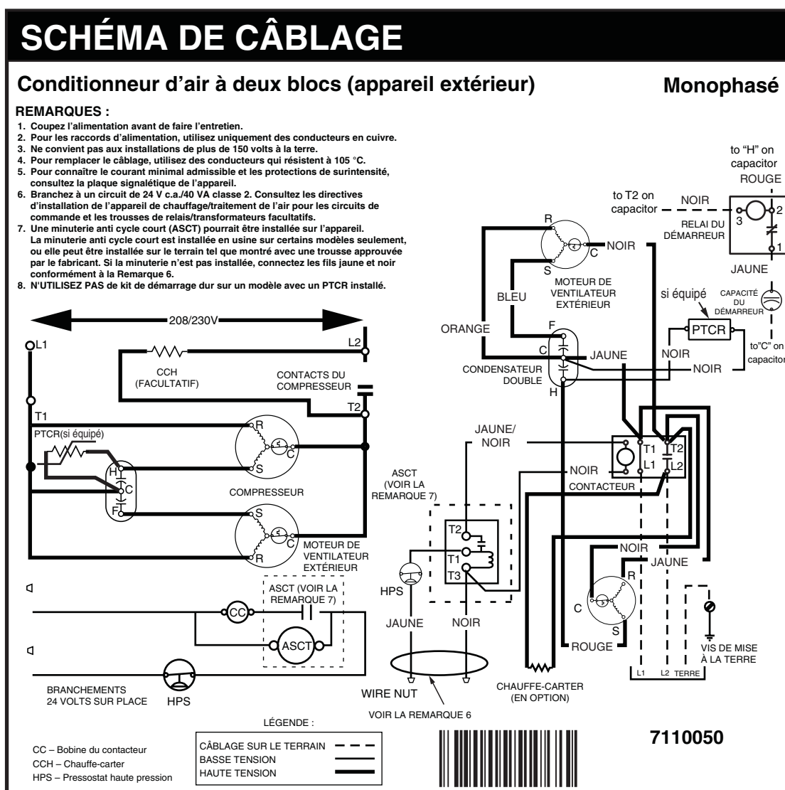
Figure 5. Schéma de câblage pour les *SA(1,2)BE4M1RN (appareils de 1,5, 2, 2,5, 3, 3,5, 4 et 5 tonnes sans le Coresense™)
