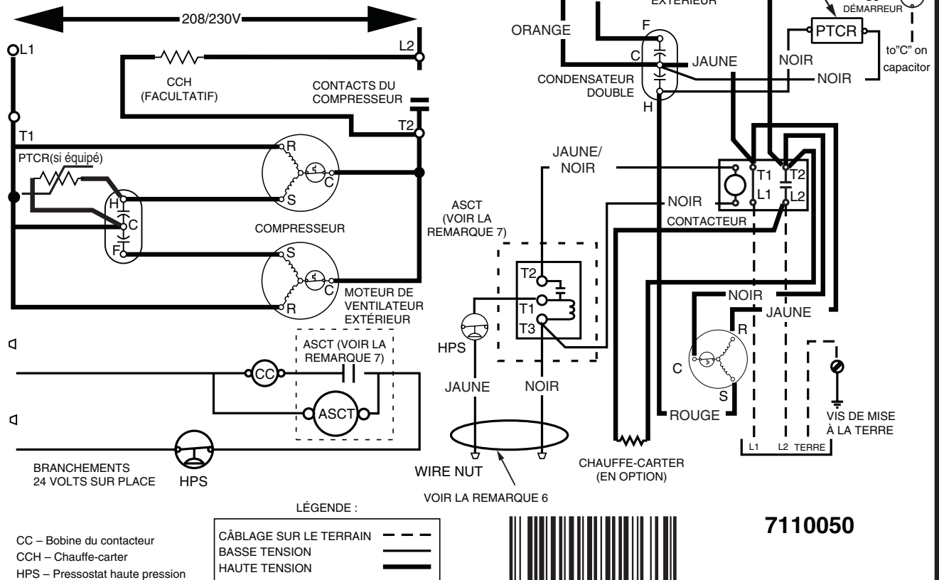
Figure 4. Schéma de câblage pour les *SA(1,2)QE4M1RN (appareils de 2, 2.5, et 3 tonnes)
