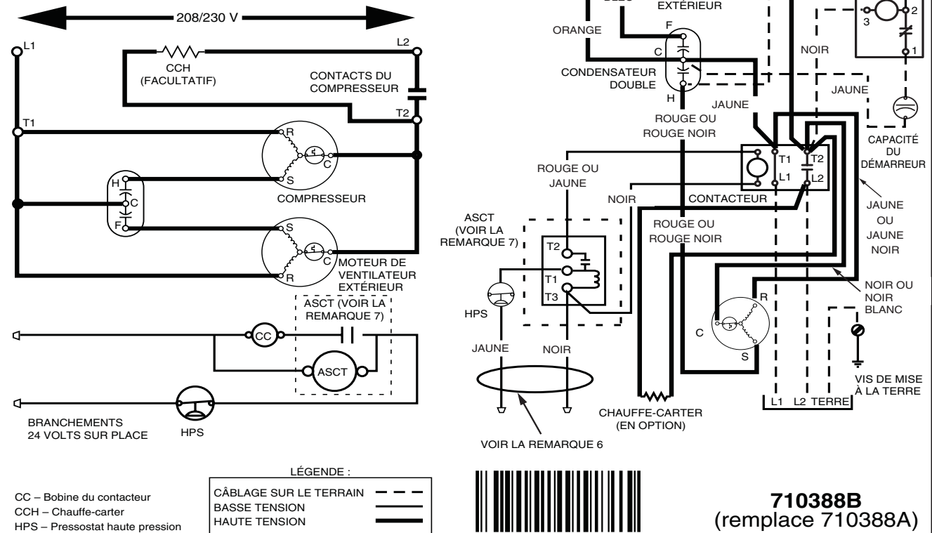
Figure 5. Schéma de câblage pour les *SA(1,2)QE4M1SN (appareils de 2, 2.5, 3, 3.5 et 4 tonnes)
