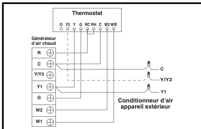
Figure 2. Conditionneur d'air bi-étages typique (sans CoreSense™) avec fournaise au gaz
