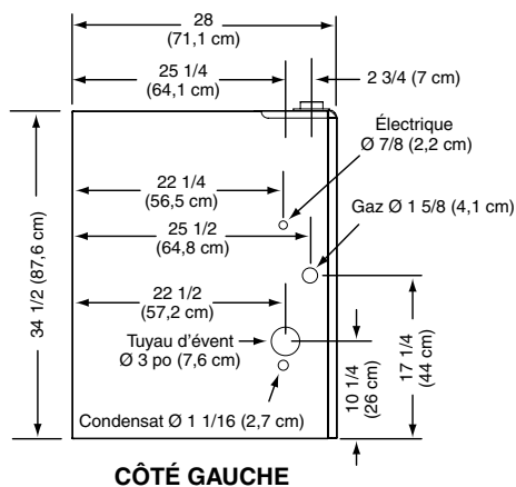
Figure 26. Dimensions des armoires *TE et *TN
