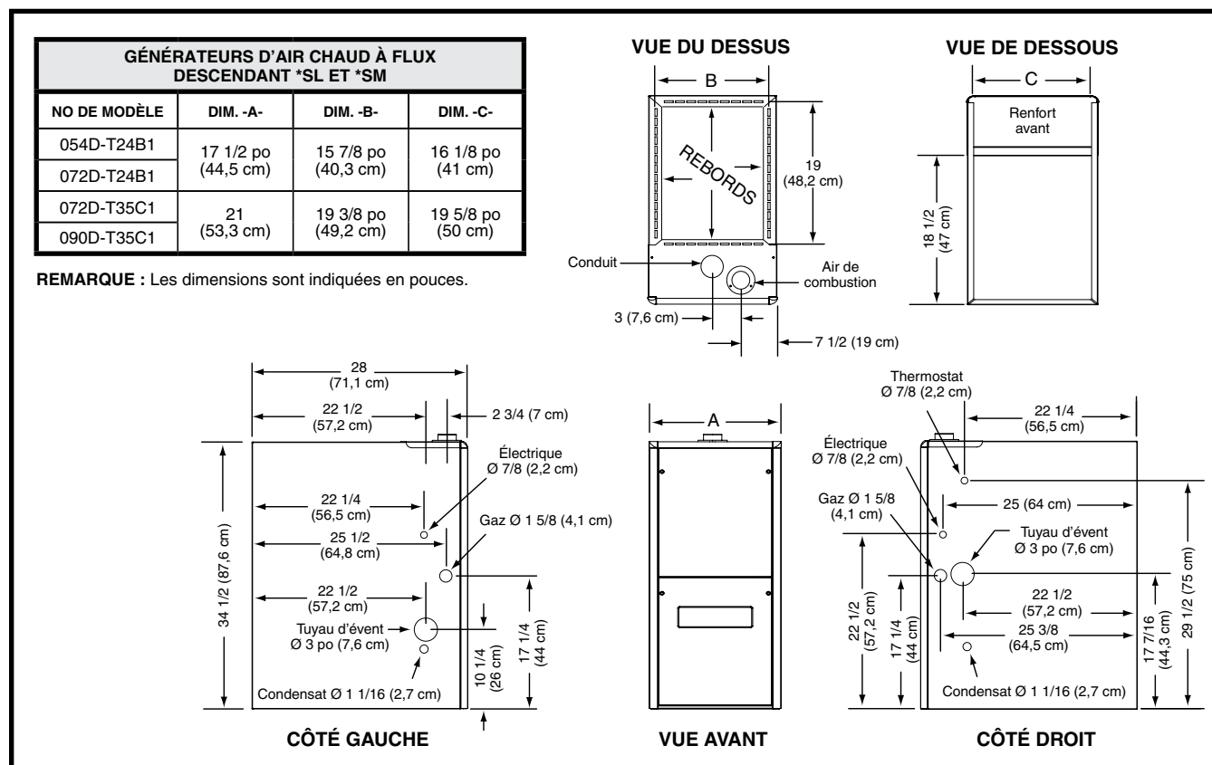
Figure 30. Dimensions des armoires *SL et *SM
