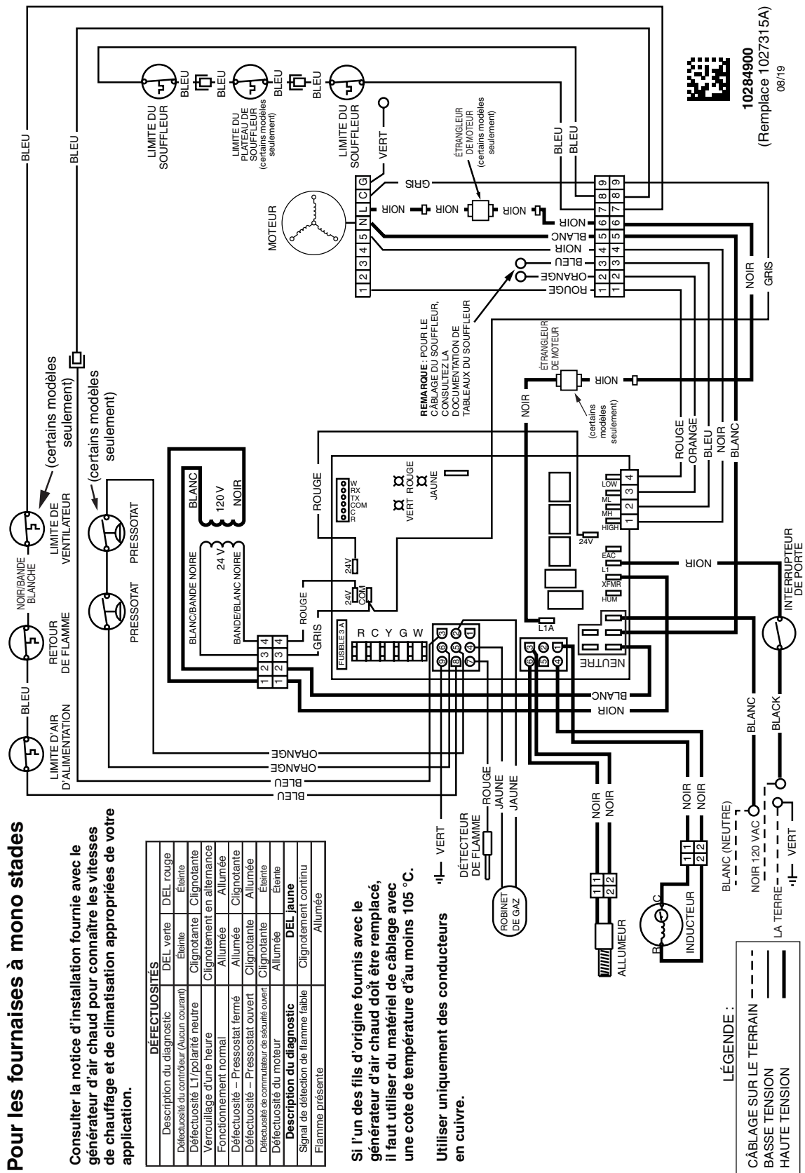
Figure 32. Schéma de câblage
