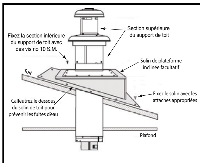
Figure 21. Toit incliné
