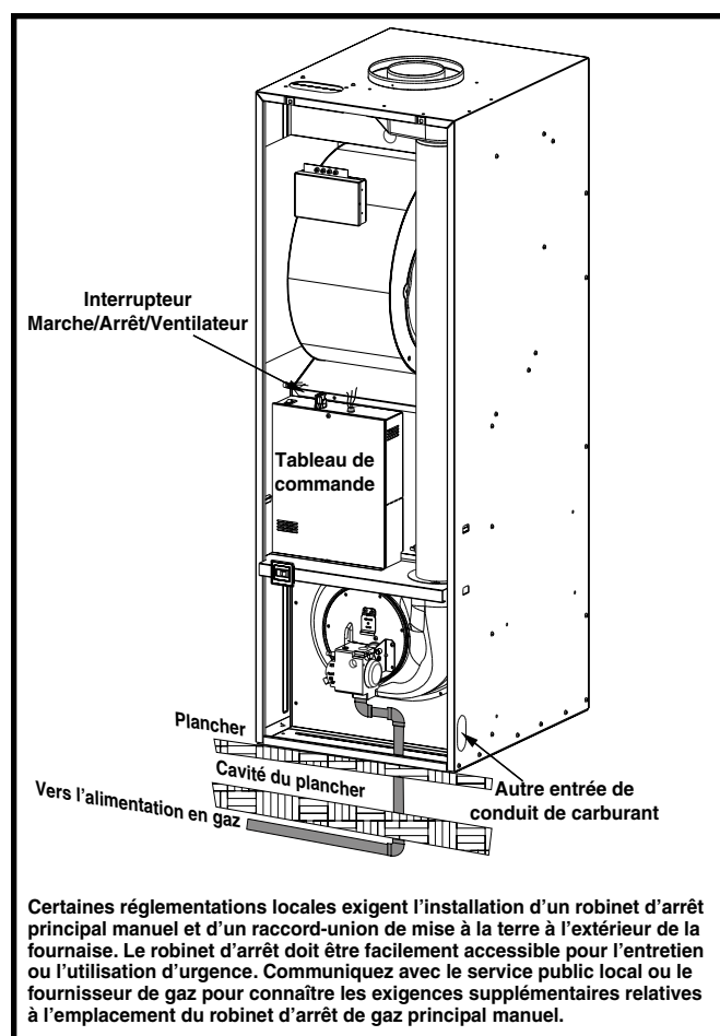
Figure 26. Tuyauterie typique de gaz
