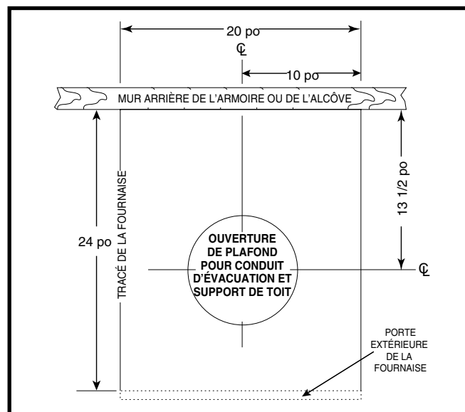
Figure 16. Dimensions de coupe pour le conduit d'évacuation et le support de toit
