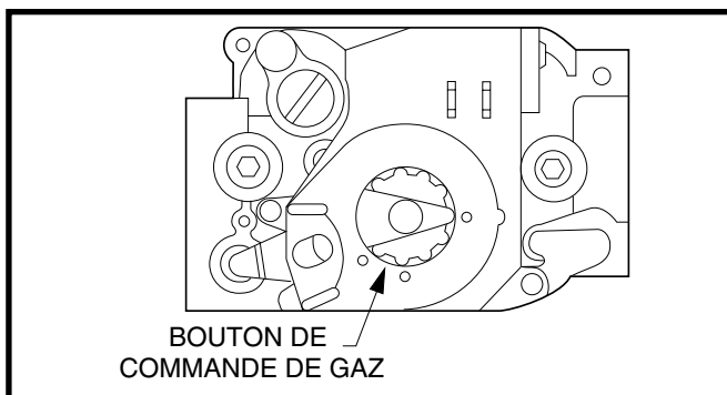
Figure 28. Robinet de gaz à allumage direct – Honeywell
