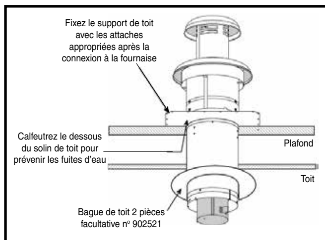
Figure 20. Toit plat
