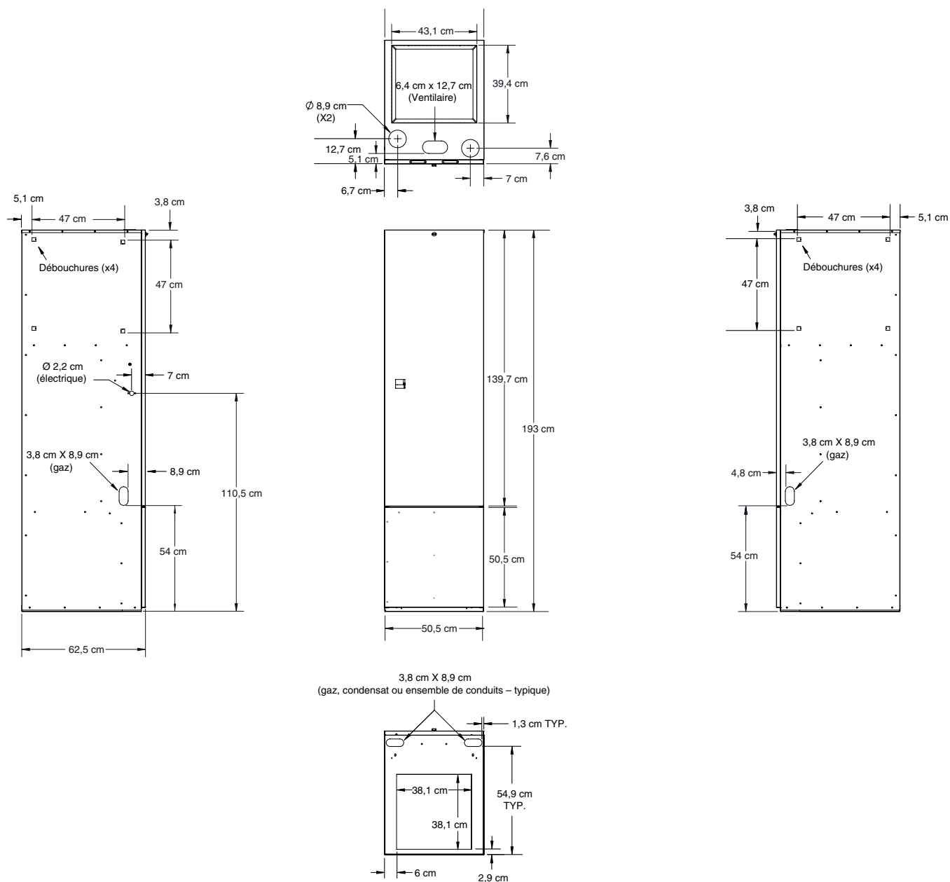
Figure 24. Dimensions modèle à reprise par le haut
