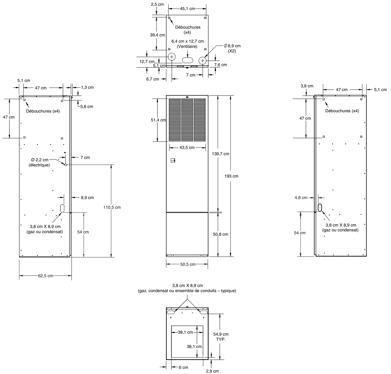
Figure 23. Dimensions modèle à reprise avant
