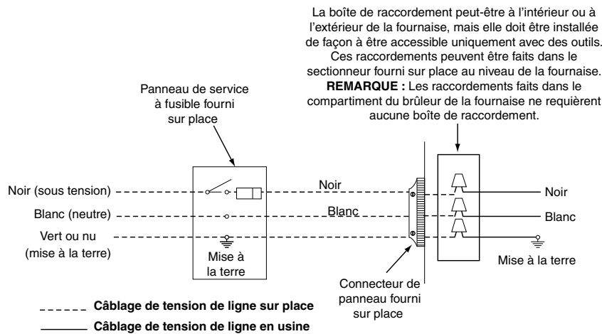
Figure 25. Câblage d'excitation de tension de ligne
