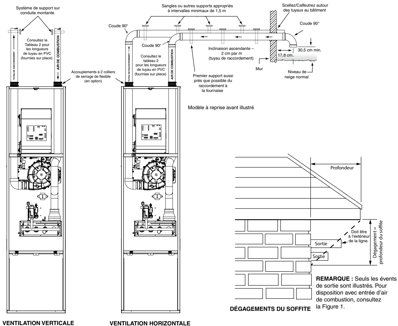
Figure 29. Évacuation horizontale/verticale et dégagements du soffite
