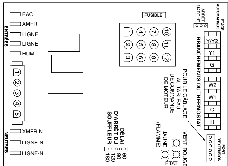
Figure 27. Tableau de commande de fournaise à deux étages
