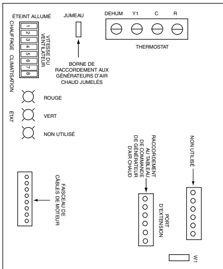
Figure 26. Tableau de commande de moteur MG2S
