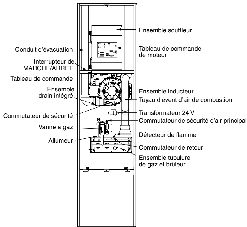
Figure 3. Composants des fournaies MG2S
