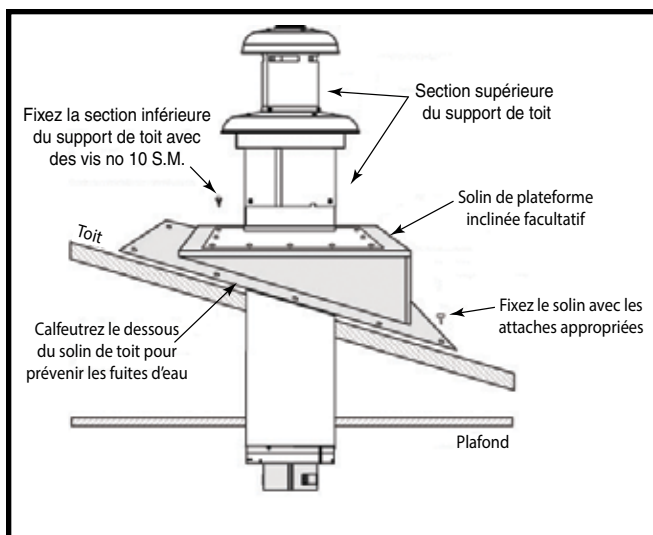
Figure 21. Toit incliné
