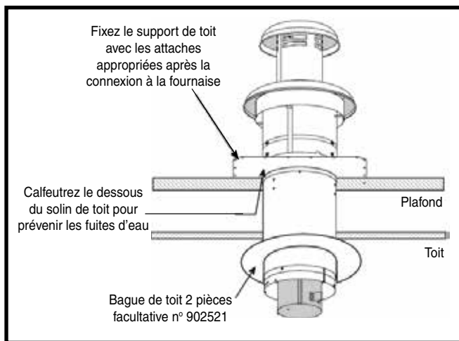
Figure 20. Toit plat
