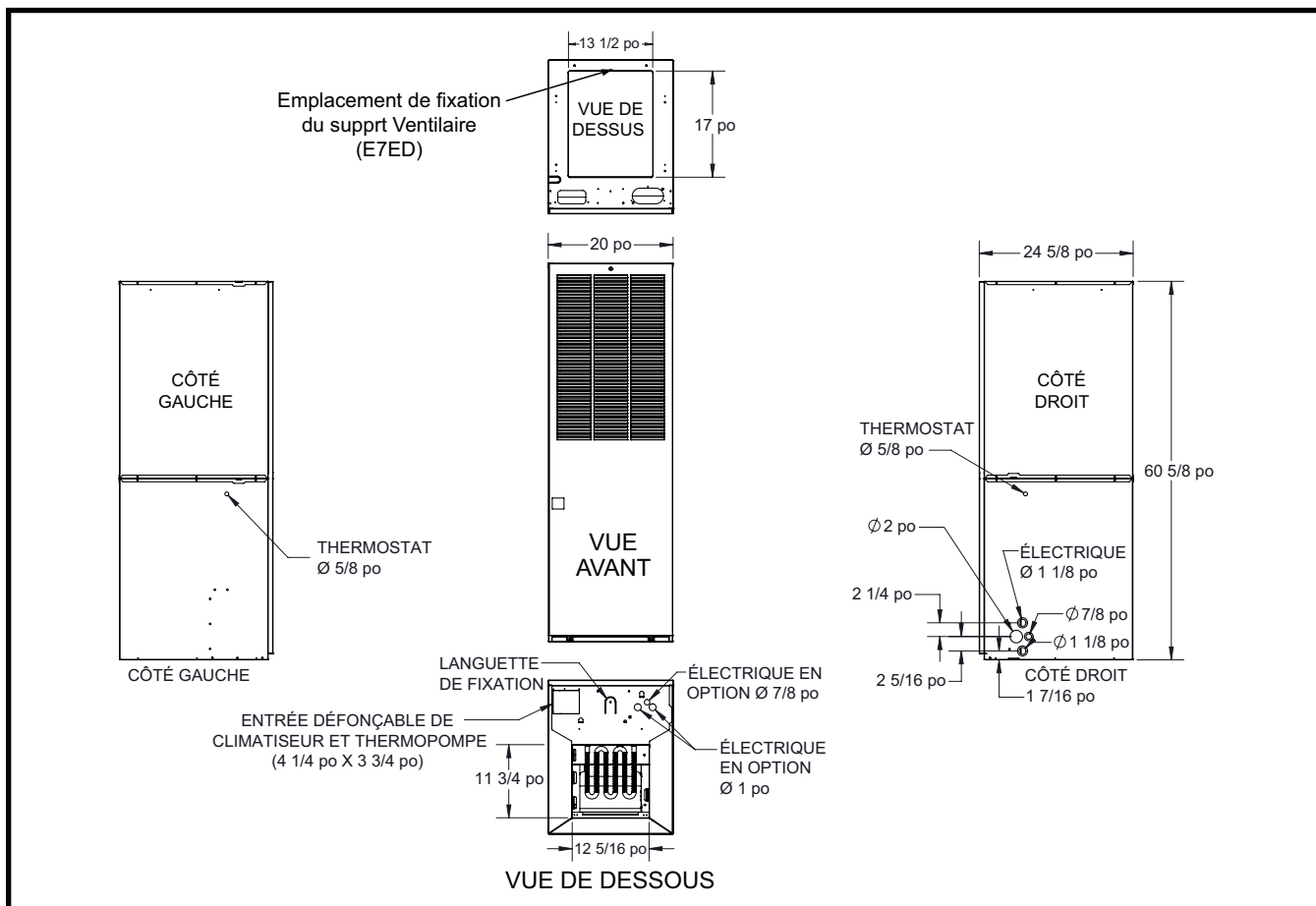
Figure 18. Dimensions de la fournaise E7EU et E7ED
