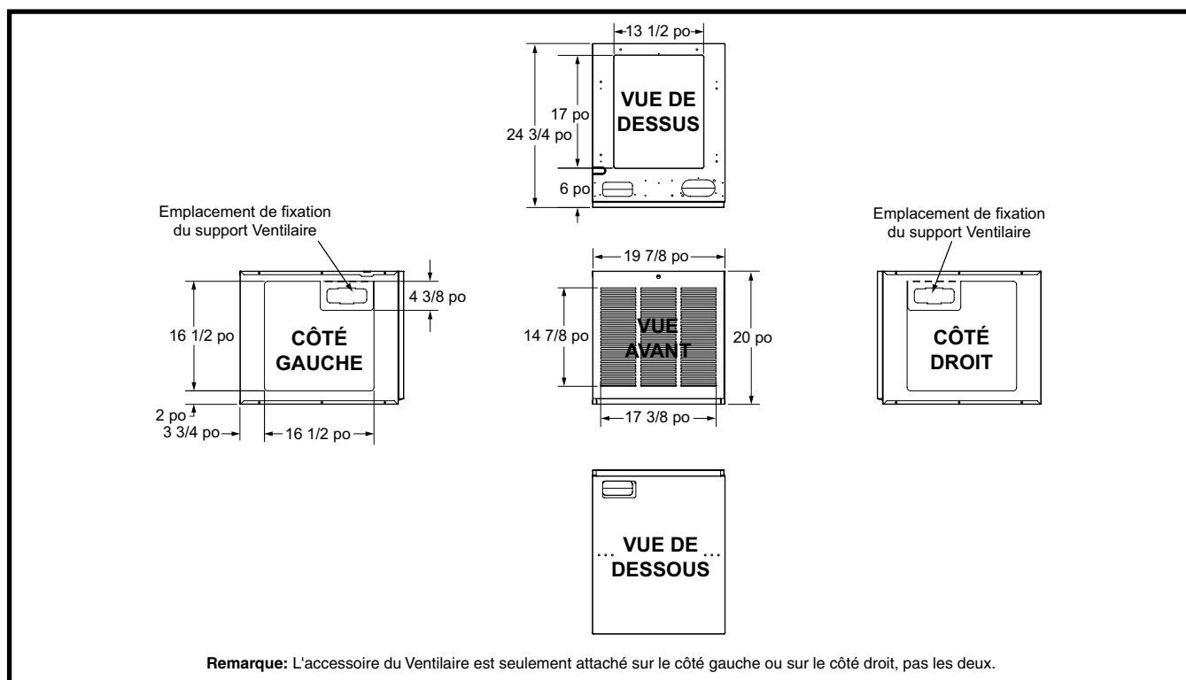
Figure 19. Dimensions du support ascendant de la fournaise E7
