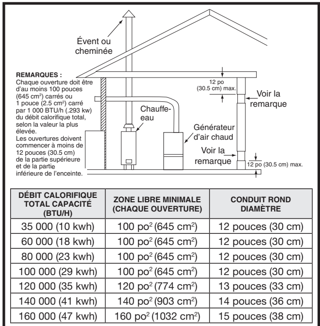
Figure 2. Air de combustion provenant de l'intérieur
