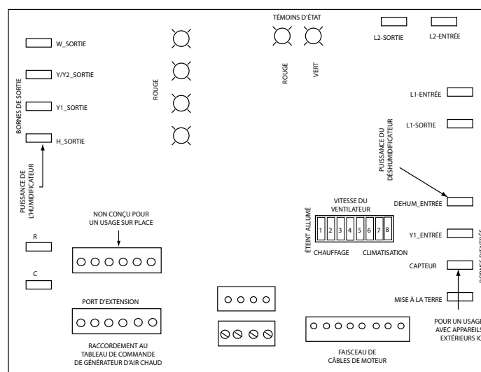
Figure 30. Tableau de commande de moteur à vitesse variable à deux étages
