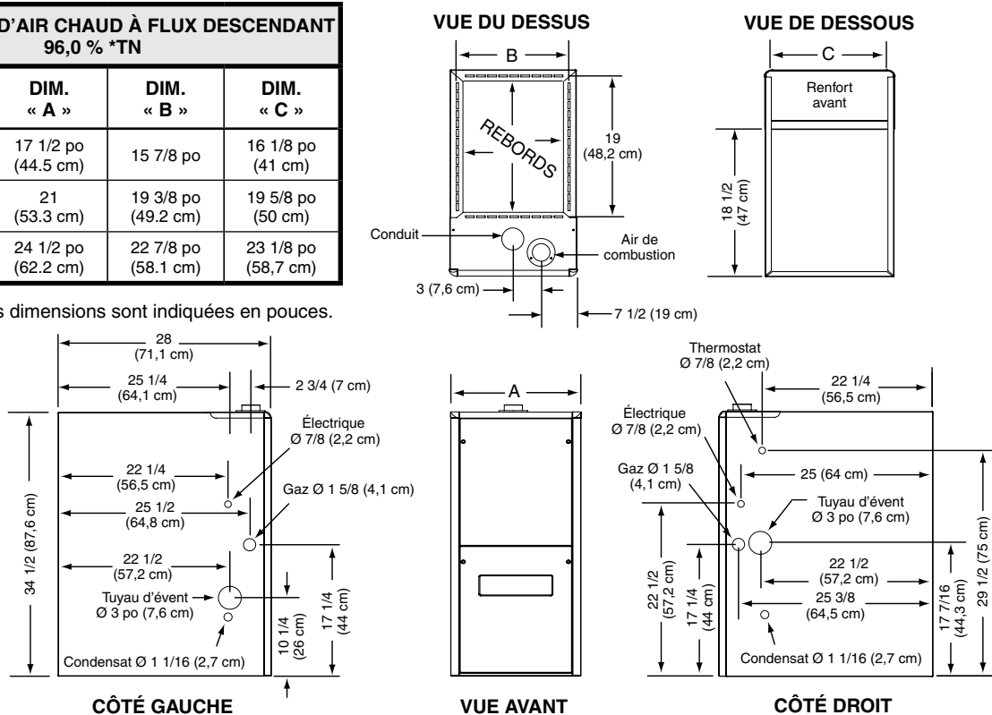
Figure 28. Dimensions des armoires *TE et *TN
