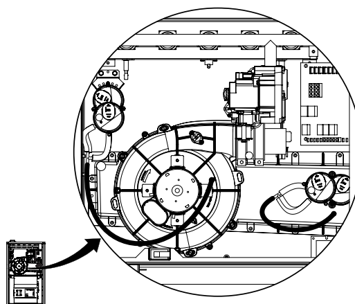
Figure 14. Tube de pressostat pour *TE générateurs d'air chaud (armoires de largeur «B», «C» et «D» seulement)
