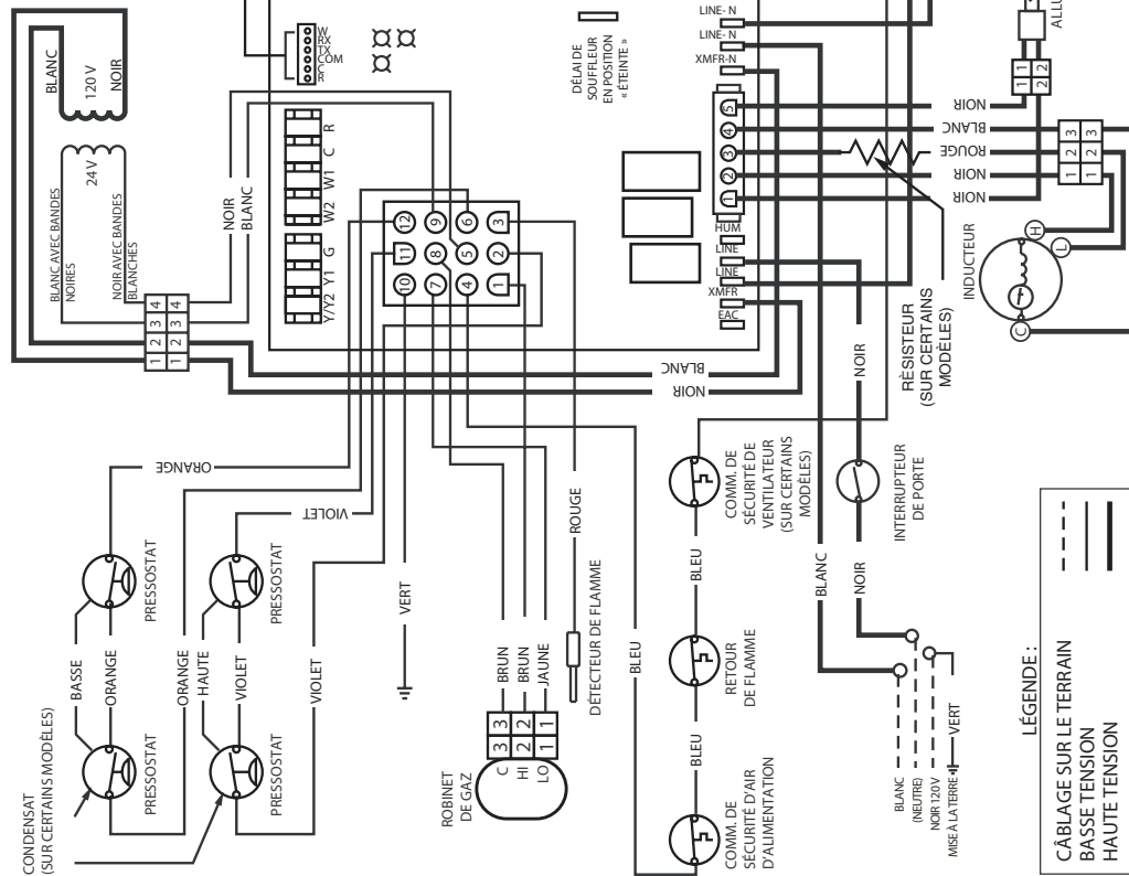
Figure 34. Schéma de câblage pour générateur d'air chaud à flux ascendant, vitesse variable et deux étages
