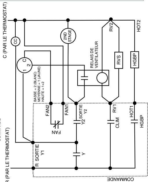
Figure 9. Schéma de câblage pour la série *SH3BE4M2XP60K (5 tonnes)
