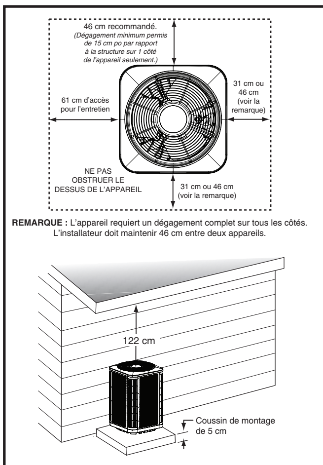
Figure 1. Dégagements requis
