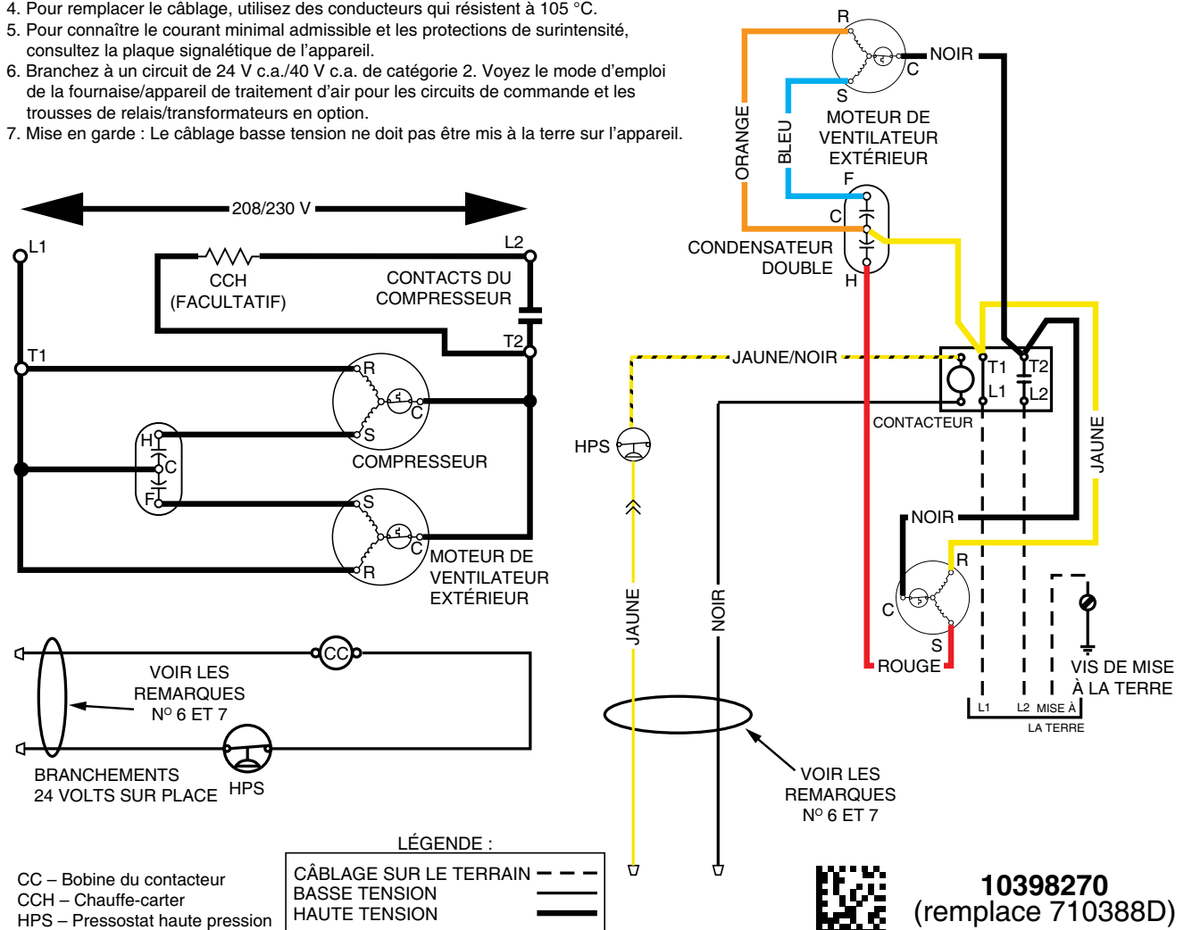
Figure 5. Schémas de câblage pour la série *SA3BD4M (modèles de 1,5 à 4 tonnes)
