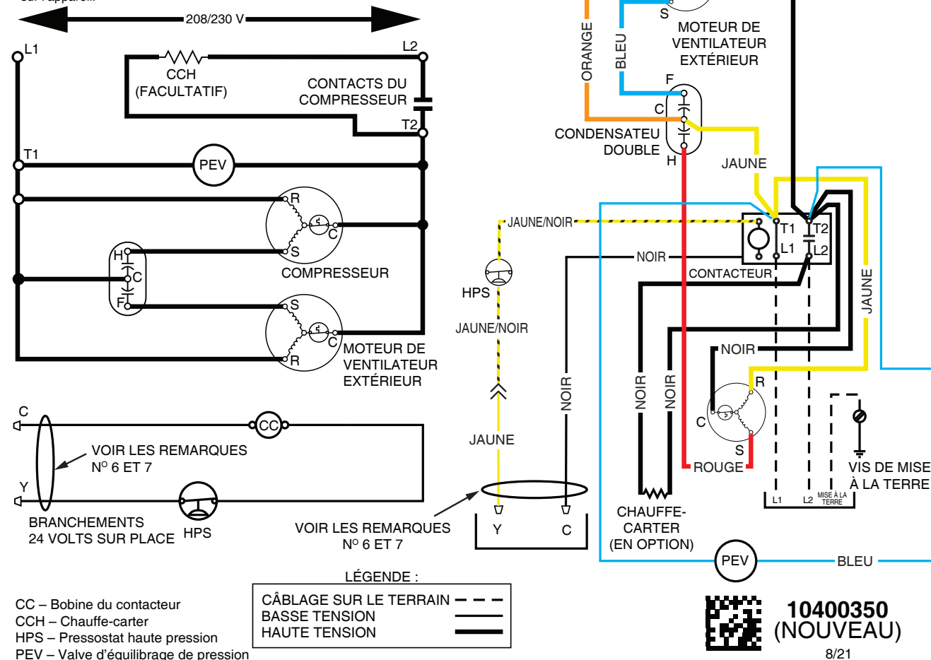
Figure 5. Schéma de câblage *SA3MD4M1RN
