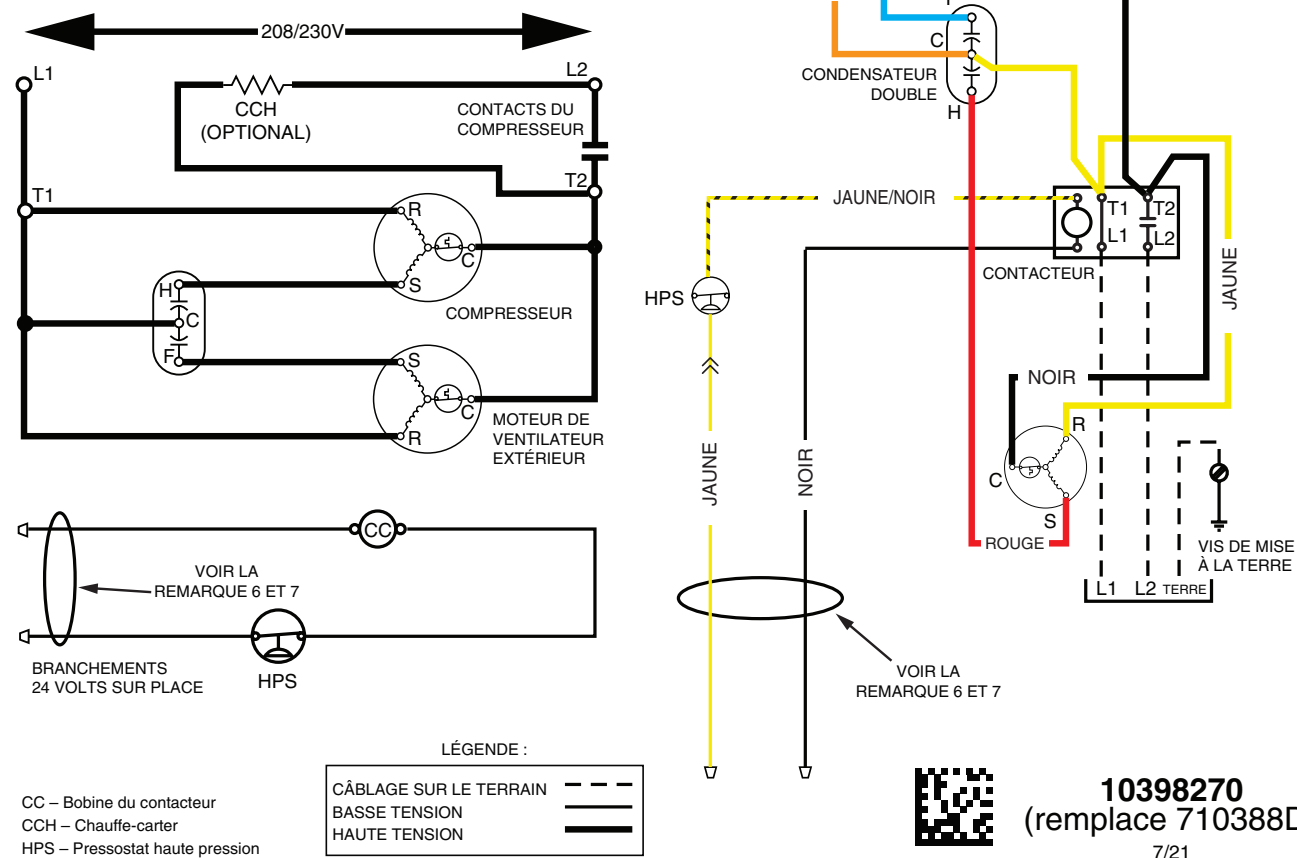
Figure 4. Schéma de câblage *SA3MD4M1SN
