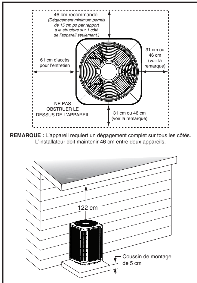
Figure 1. Dégagements requis
