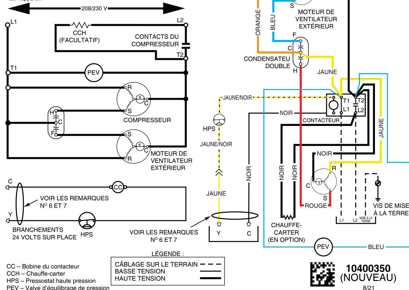
Figure 6. Schéma de câblage pour le *SA3QD4M1RN
