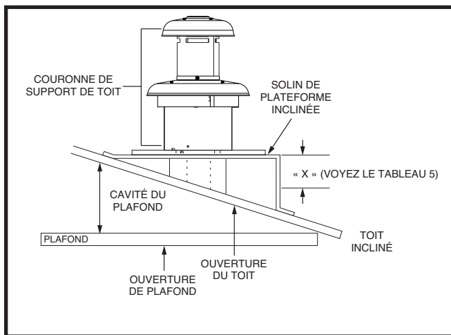
Figure 18. Exemple de support plat avec solin
