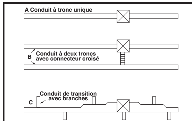
Figure 6. Système de conduit d'alimentation typique
