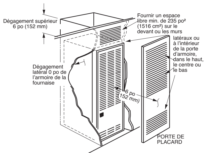
Figure 2. Installation dans un placard
