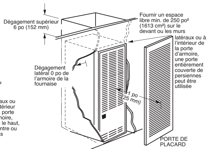
Figure 1. Installation dans une alcôve
