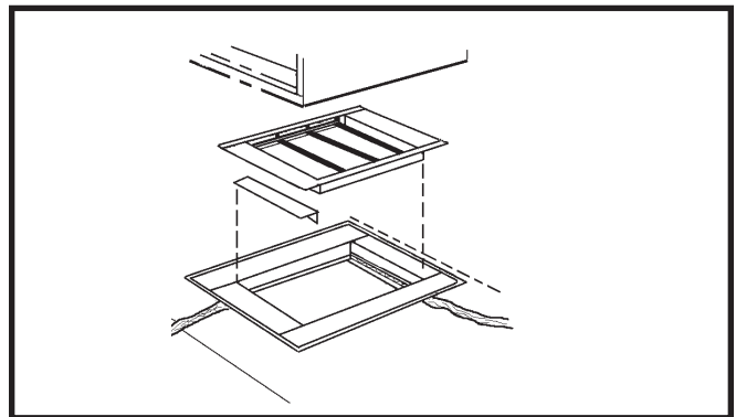
Figure 32. Sans registre de cavité à serpentin
