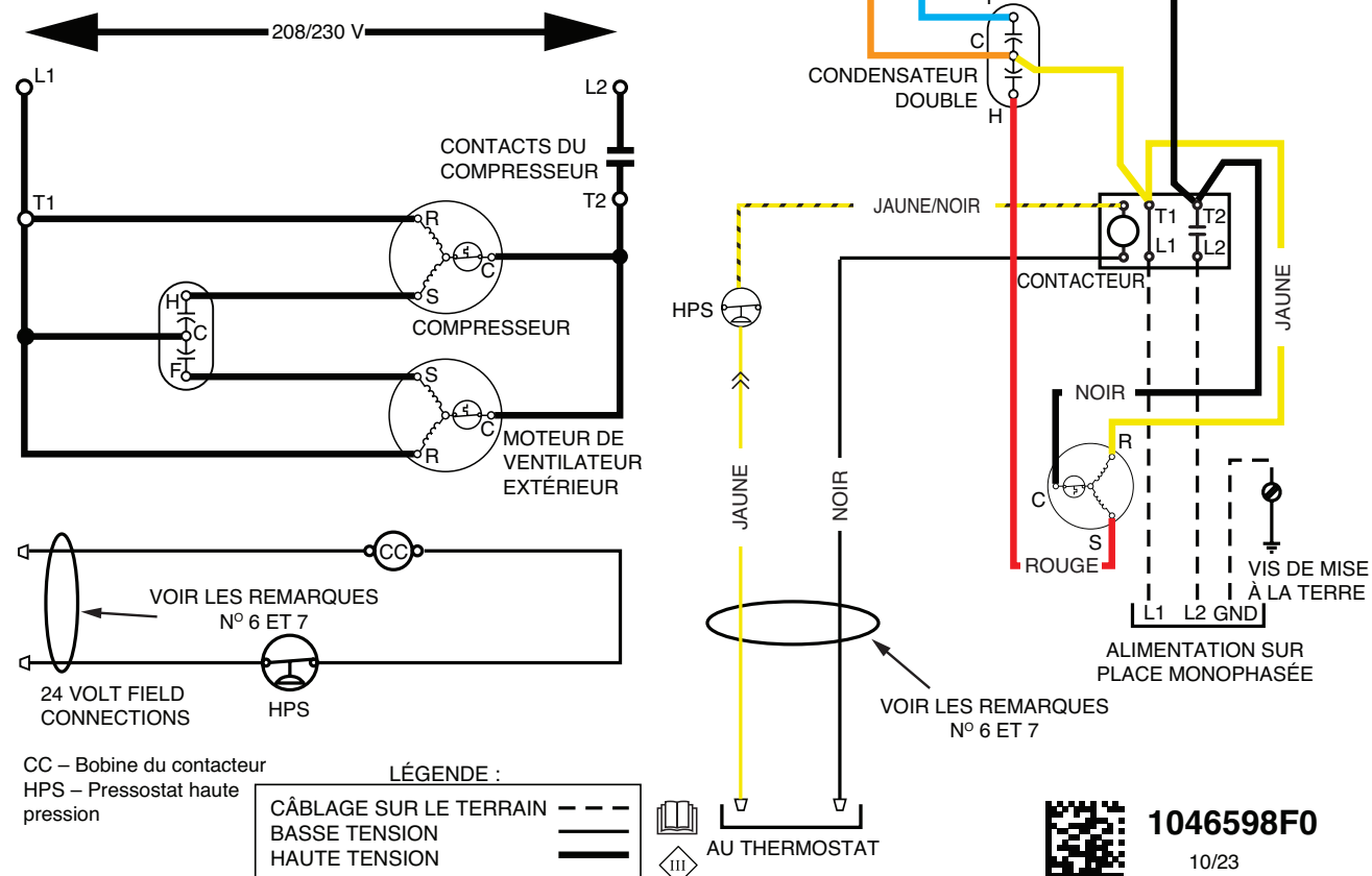
Figure 4. Schémas de câblage pour la série *SA4ME5M1SN (modèles de 2, 2,5, 3, 3,5, 4 et 5 tonnes)
