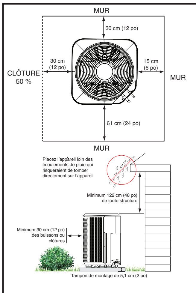
Figure 1. Dégagements requis
