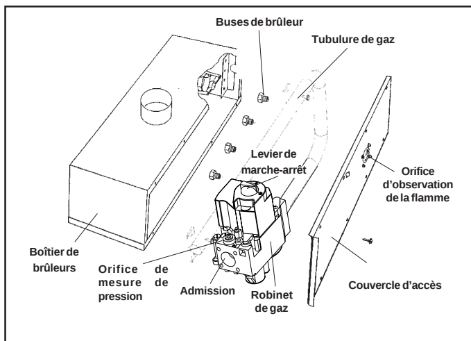
Figure 2 - Boîtier de brûleur scellé typique avec couvercle d'accès
