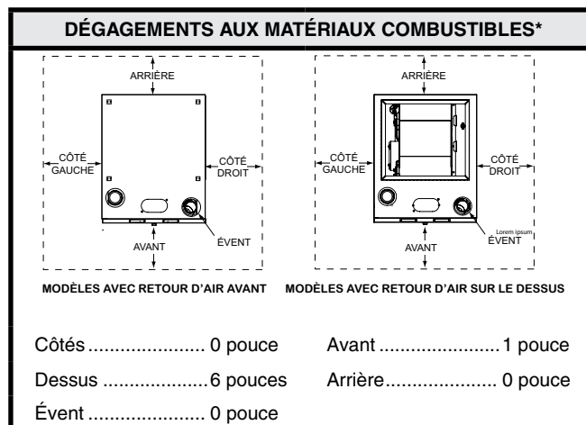
Figure 1. Dégagements minimaux
