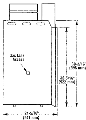
Left Side
